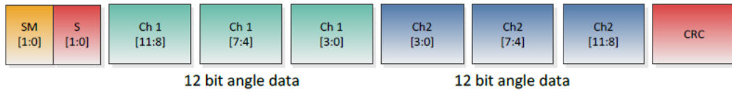
图13 A.1双阀体位置传感器数据帧
