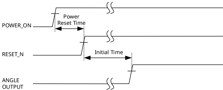
图7 上电复位时序
