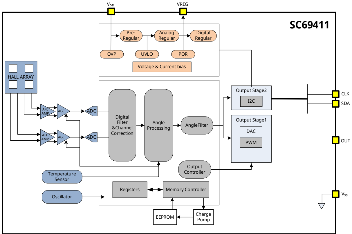
图9 功能框图
