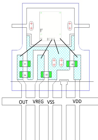
图32 SIP3 单芯片封装应用参考电路图
